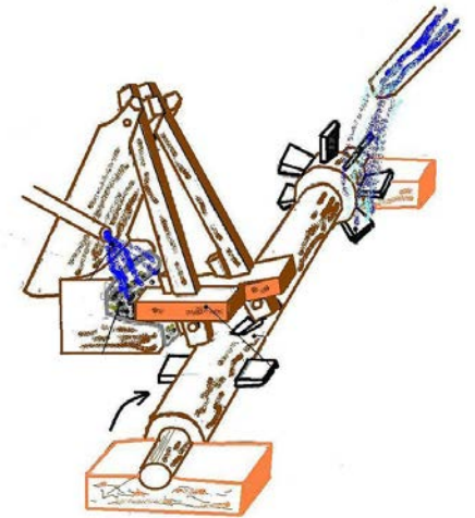
Fonctionnement du moulin
